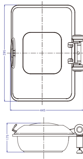
15706 スマートチューフィンゴオブロンダ (ガラス) ¥180,000 58.1×43.5×H21.0cm (8.0ℓ) 付属品: ステンレスフードパン 1/1・スプーンホルダー別売
