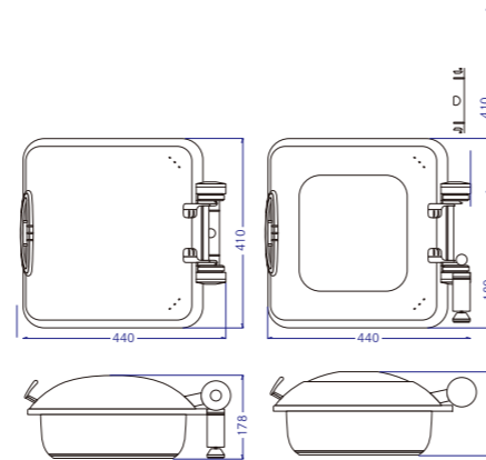
15700 角型スマートチューフィン本体 (ガラス) ¥155,000 41.0×44.0×H18.0cm (5.5ℓ) 付属品: ステンレスフードパン 2/3・スプーンホルダー別売
