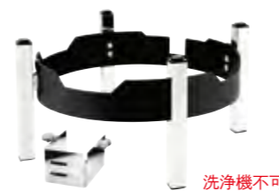
11282-000 Tチューフィンスタンド (スタッキング対応) ¥59,000 50.0×45.6×H24.4cm 付属品: パナーホルダー [対応: 15801 シリーズ]
