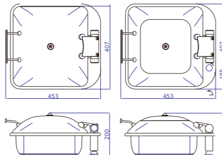
15601 角型スマートチューフィン本体 (ガラス) ¥145,000 45.3×40.7×H19.5cm (5.5ℓ) 付属品: ステンレスフードパン 2/3・スプーンホルダー別売
